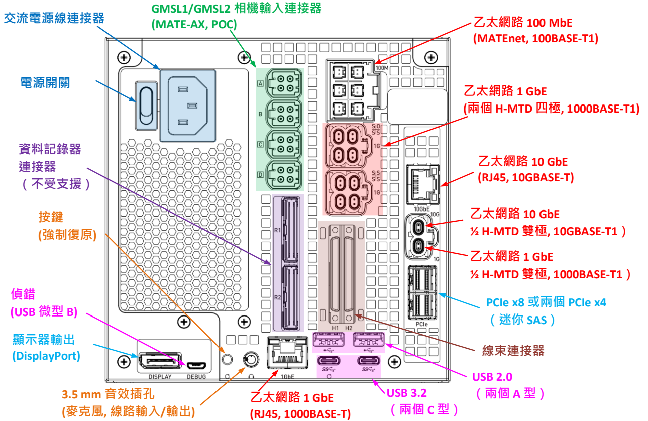
圖 2. 後面板連接器
