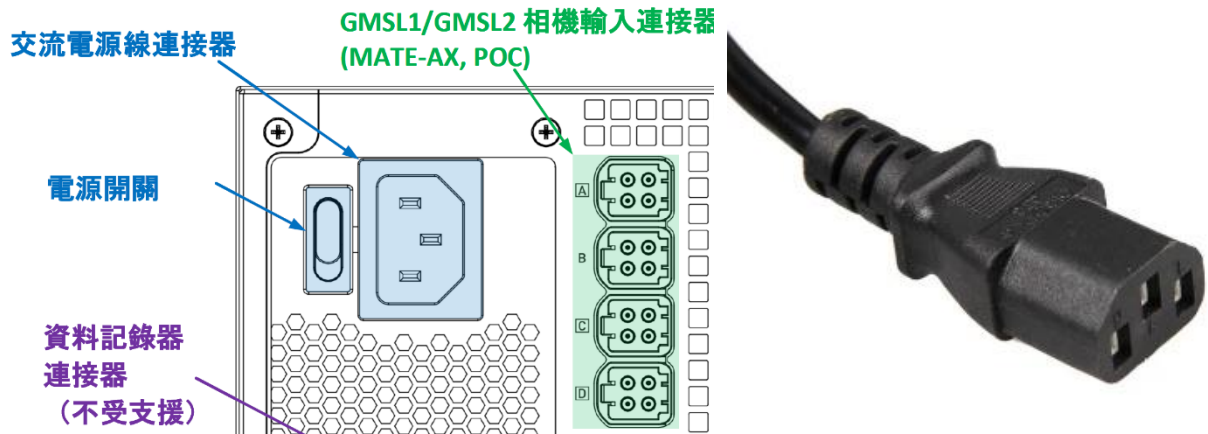
圖 3. 電源連接器和電源線
